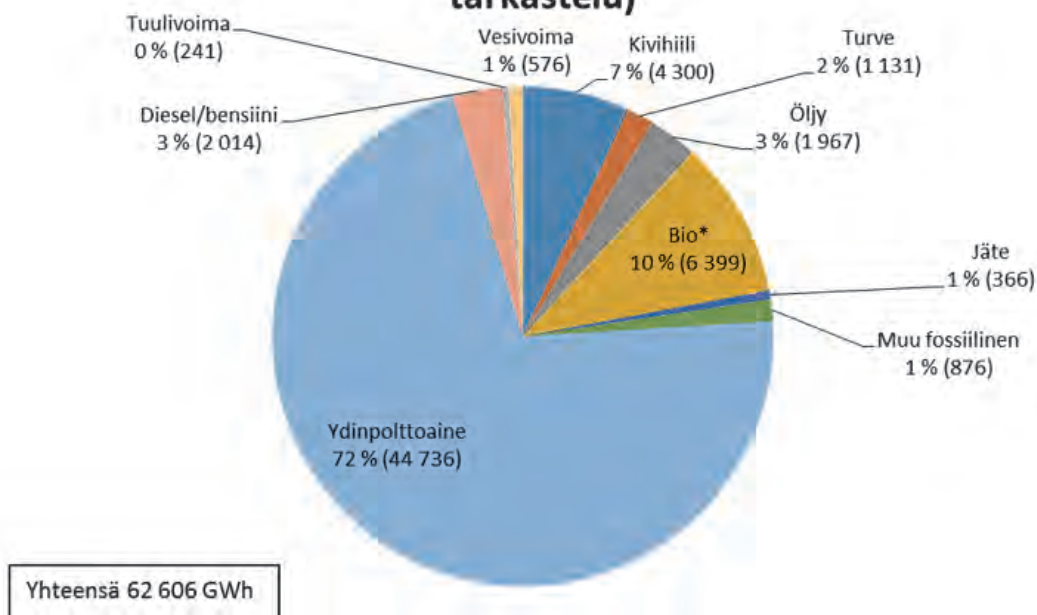
Kuva 39. Satakunnan energiantuotannon jakautuminen energialähteittäin vuonna 2014 (energiälähteiden määriin pohjautuva tarkastelu). Suluissa olevat luvut kuvaavat tietyn energialähteen energiamäärää gigawattitunteina (GWh). * = Luokka Bio tarkoittaa biopolttoaineita, joita ovat kaikki puupohjaiset polttoaineet.
