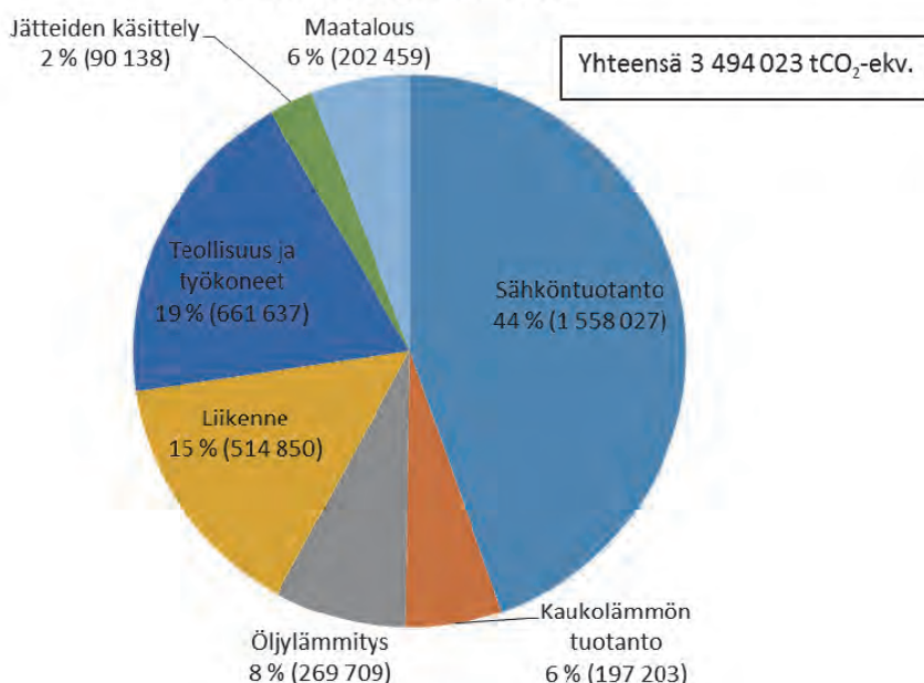
Kuva 42. Satakunnan alueperusteisten kasvihuonekaasupäästöjen jakautuminen vuonna 2014. Suluissa olevat luvut kuvaavat tietyn päästöluokan päästöjä hiilidioksidiekvivalenttitonneina (tCO 2 -ekv). Liikenne-päästöluokka ei sisällä lentoliikenteen päästöjä.
