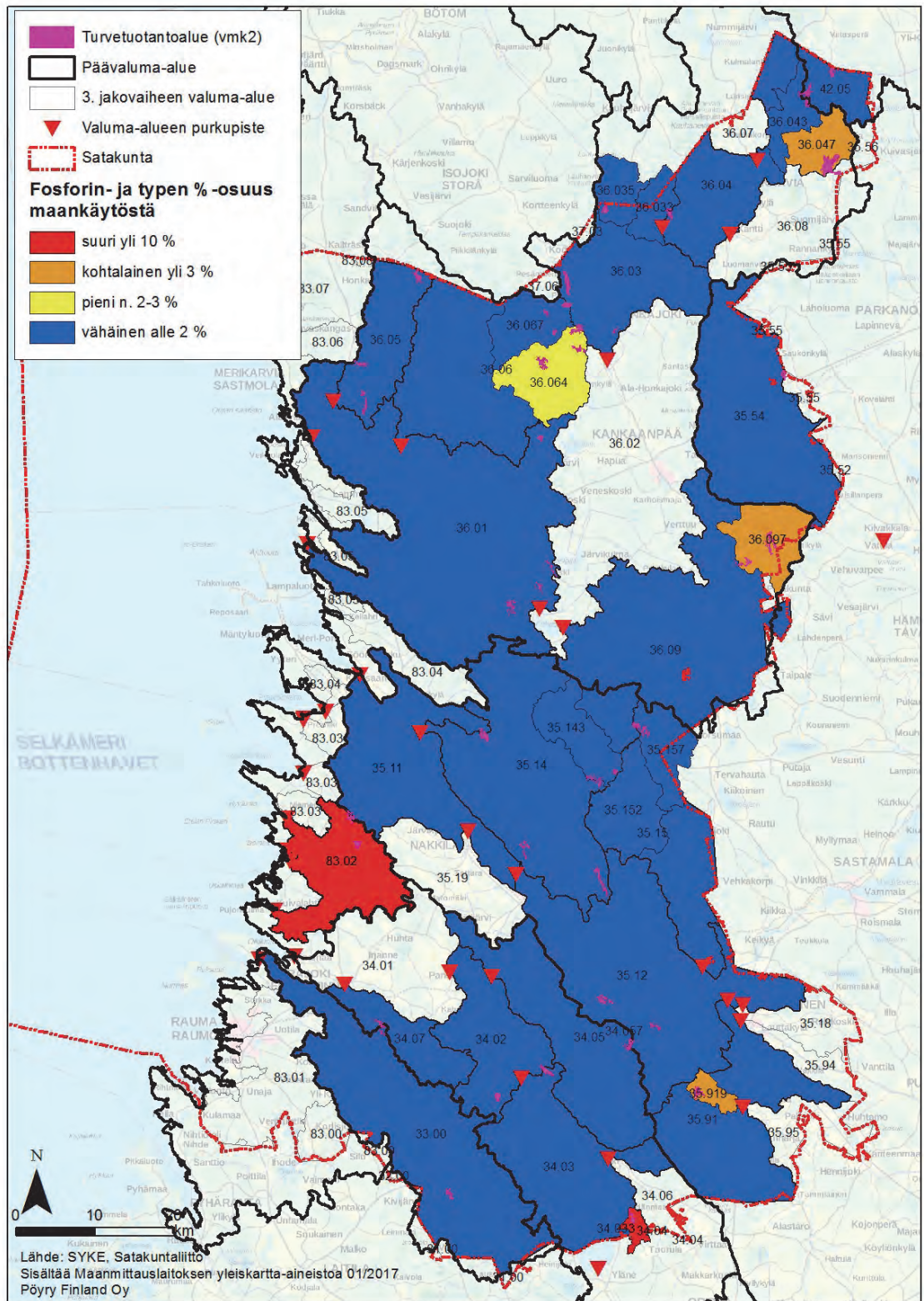
Kuva 48. Satakunnan vaihemaakuntakaavan 2 valmisteluvaiheen aineistossa osoitettujen turvetuotantoalueiden kuormituksen (fosfori ja typi) prosenttiosuus kaikesta maankäytöstä.
