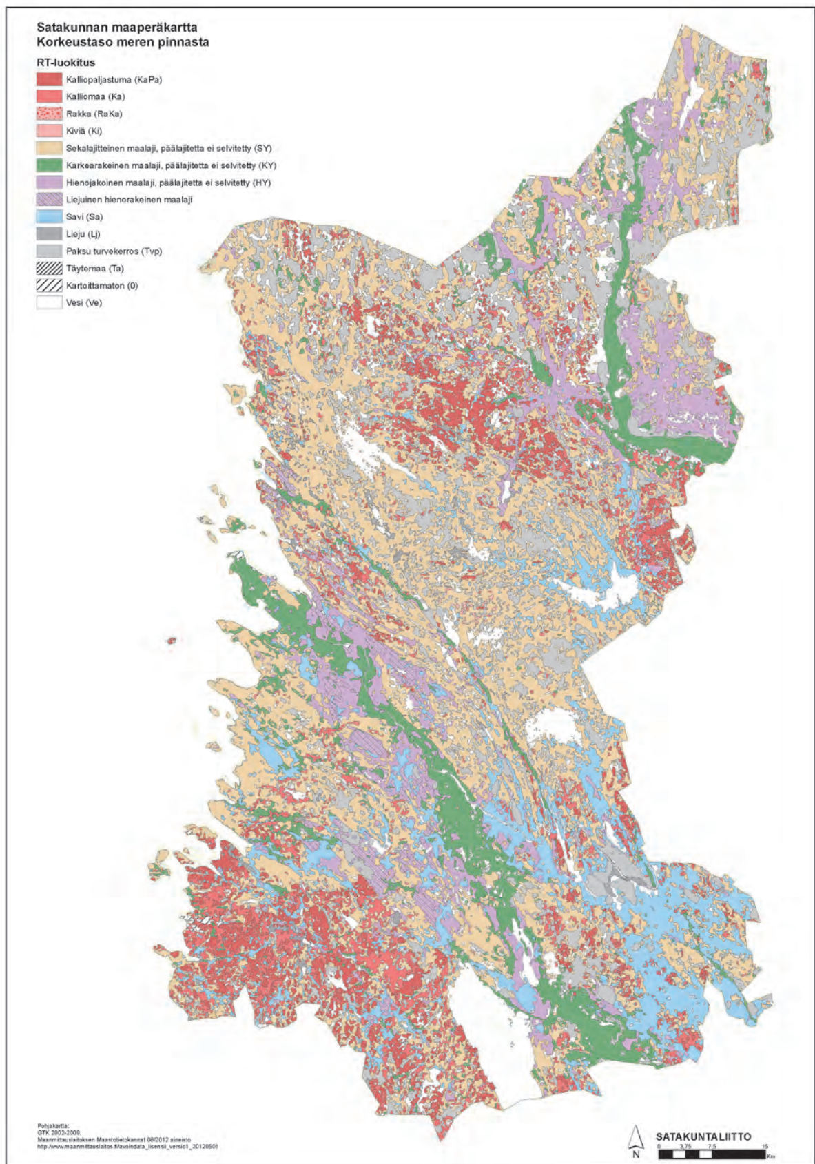
Kuva 6. Satakunnan maaperä. 12
