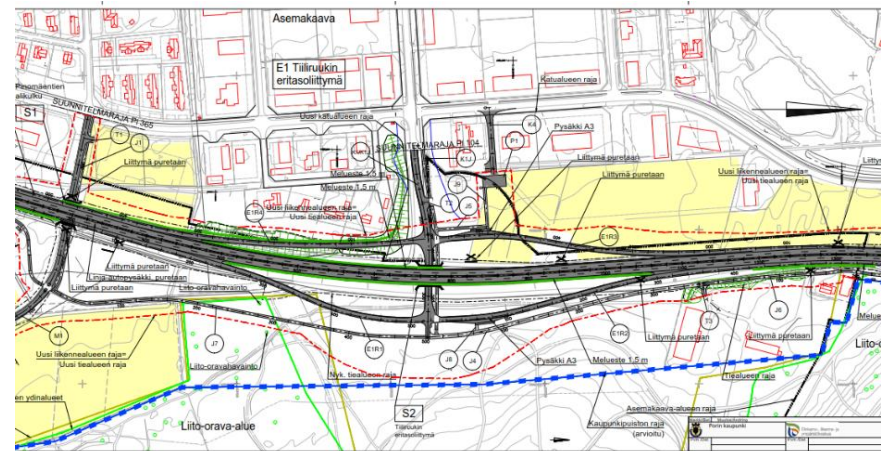
Vt 8 Tiiliruukin eritasoliittymän aluevaraussuunnitelma, vaihtoehdot 3 ja 4 (Porin kaupunki)
