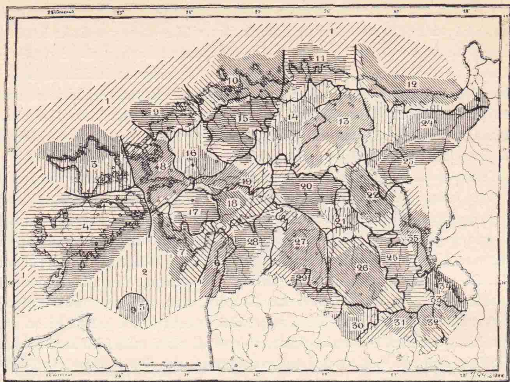
Piirr. 34. Viron maantieteelliset kolmen ja neljän aineksen seudut sekä ensinmainittuja vastaavat kuntaryhmit.
