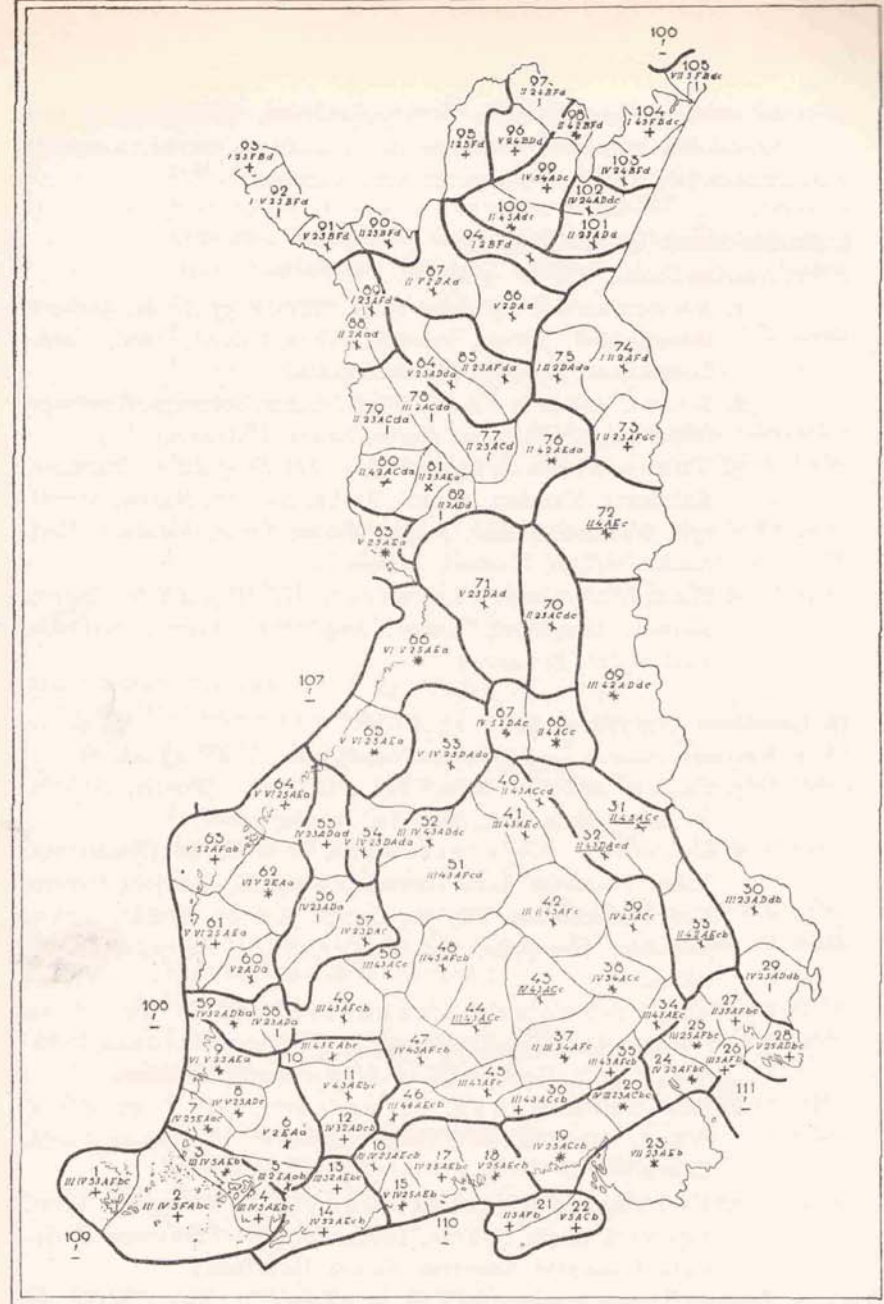
Kartta 8. Maantieteelliset seudut järjestysnumeroineen, maisemakaavoineen ja yksilöllisyysmerkkeineen.
